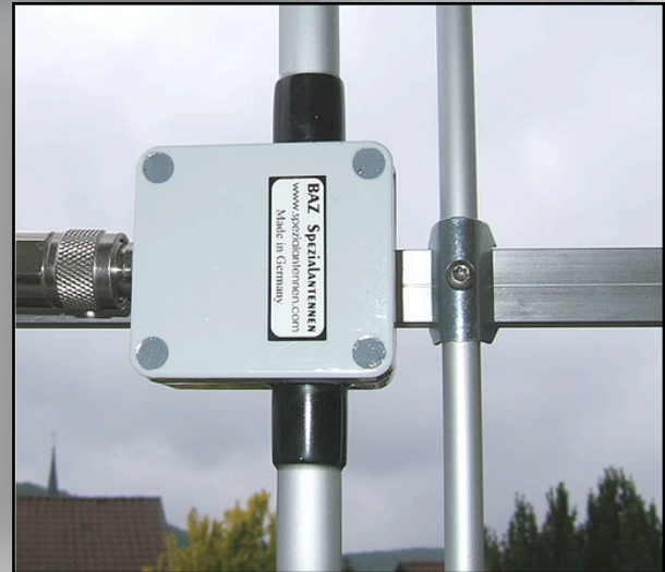
4 Element Yagi-Richtantenne
